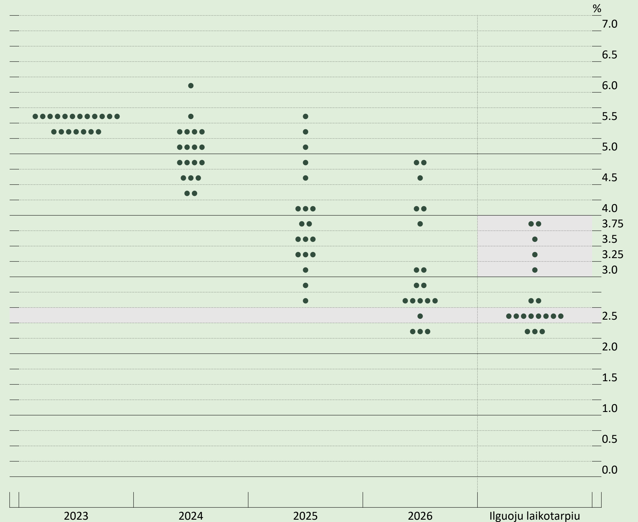
FED dot-plot palūkanų normos projekcija:**
